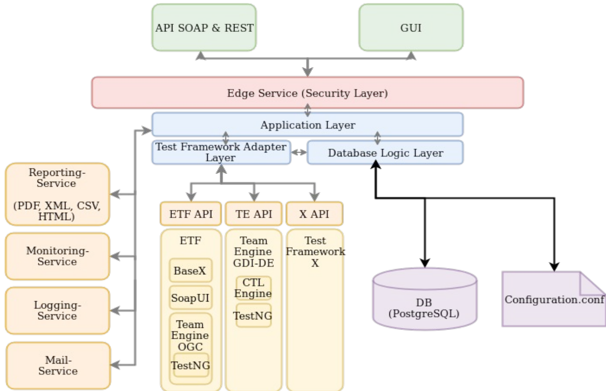
Abbildung 1: Systemarchitektur
